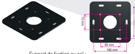
Support de fixation au sol : ST4510
